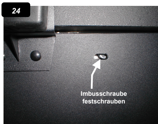
WICHTIG 24. Befestigen Sie die Plasmameinheit links u. rechts jeweils 2x am Grundgestell. Die Schrauben (4x) sind bereits am Plasma angebracht.
