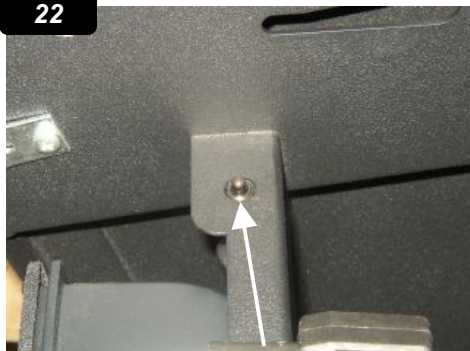
22. Ziehen Sie die Plasmasicherung nach unten, um das Plasma nach hinten zu bekommen.
