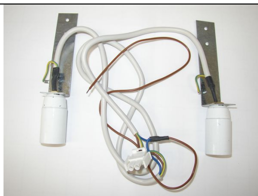
360.110.790 Kabelbaum Kerzenlampen SB MAX PRO
